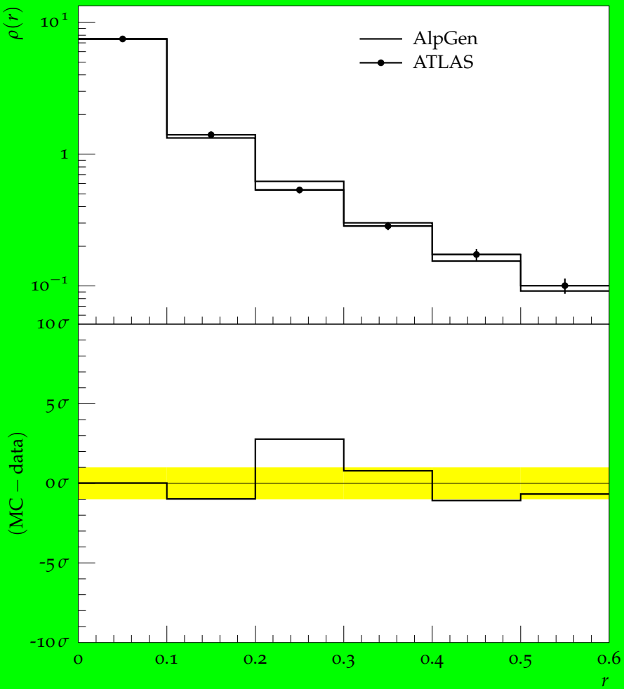
Jet shape \rho for p_{\perp} \in 310\text{--}400\text{GeV} , y \in 0.0\text{--}2.8
